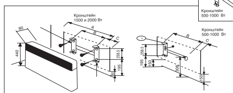
рис. 2 (размеры в мм)
